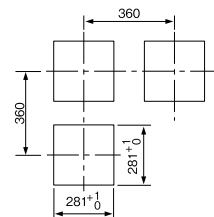
●パネルカットおよび取付最小寸法
