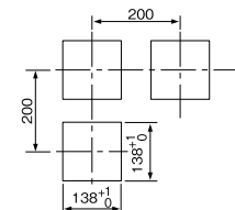
●パネルカットおよび取付最小寸法
