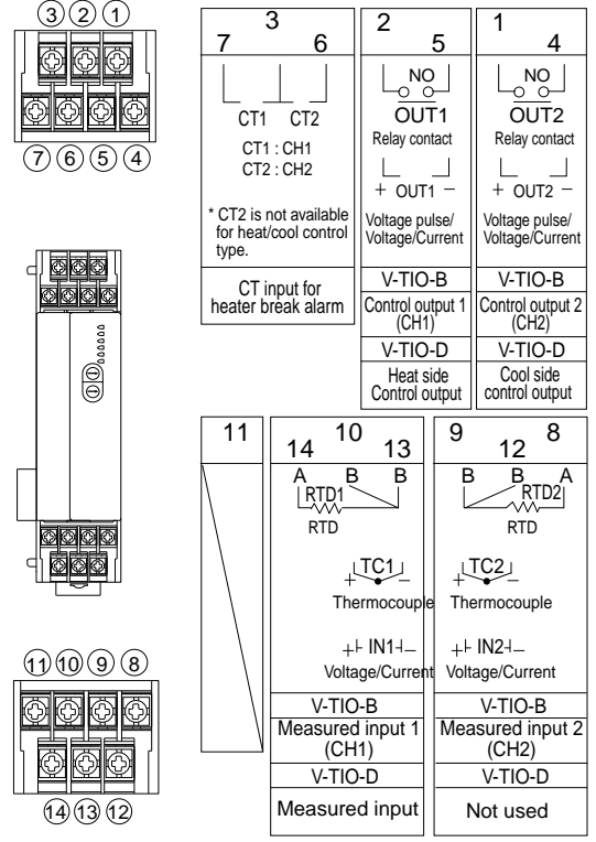
Extension Module V-TIO-B, V-TIO-D
