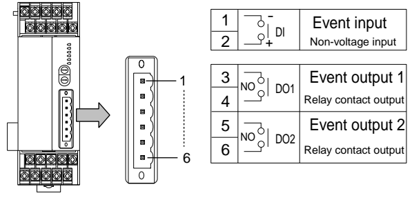
Connector (Event input/output) V-TIO-A, V-TIO-B V-TIO-C, V-TIO-D
